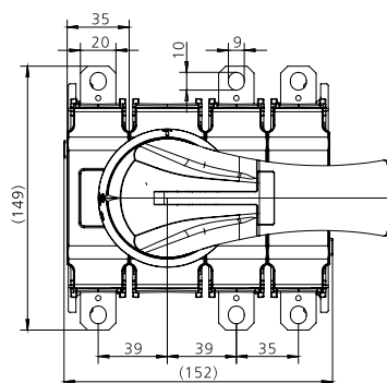
YCOT EHA C 315/250A 12
