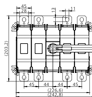
YCOT EHA B 630/630A 22
