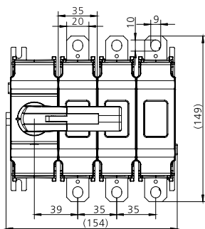
YCOT EHA B 315/250A 03
