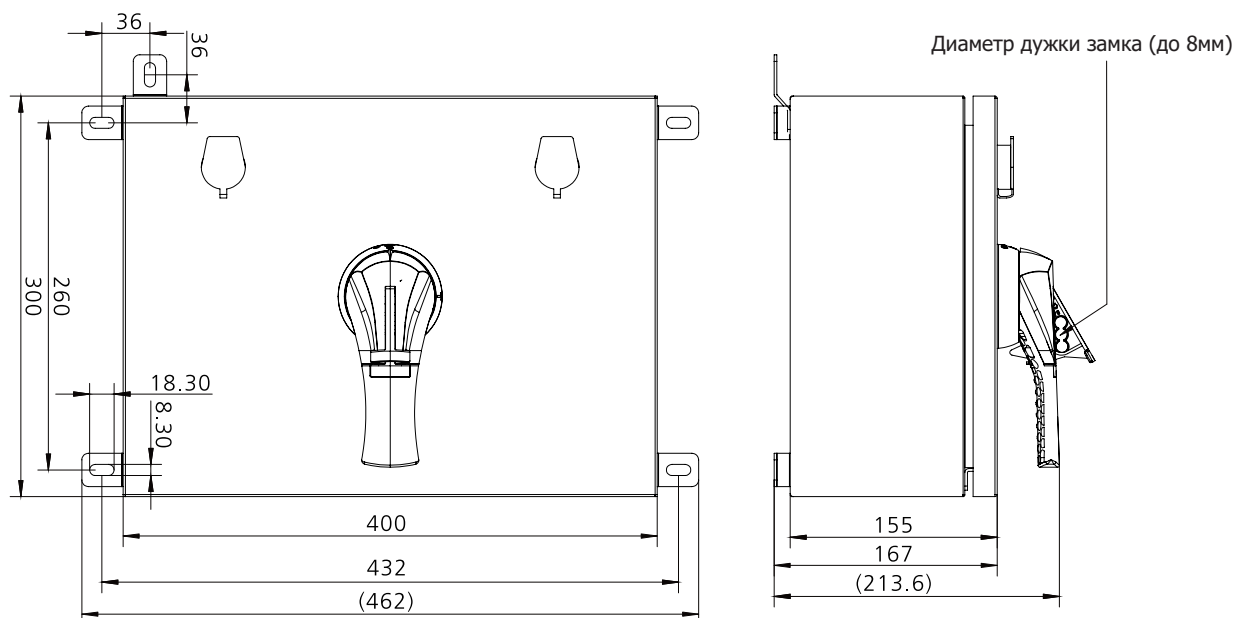
YCOT EHA M 315/250A 22
