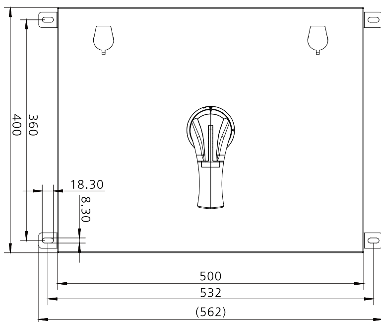
YCOT EHA M 630/630A 22
