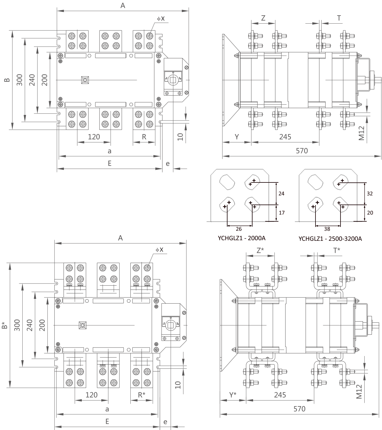
YCHGLZ1 2000-3200A с боковым управлением
