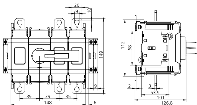
YCOT EHA C 315/250A 12
