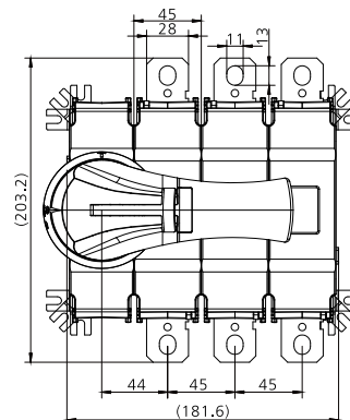
YCOT EHA C 630/800A 22
