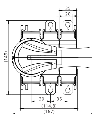
YCOT EHA C 315/250A 02
