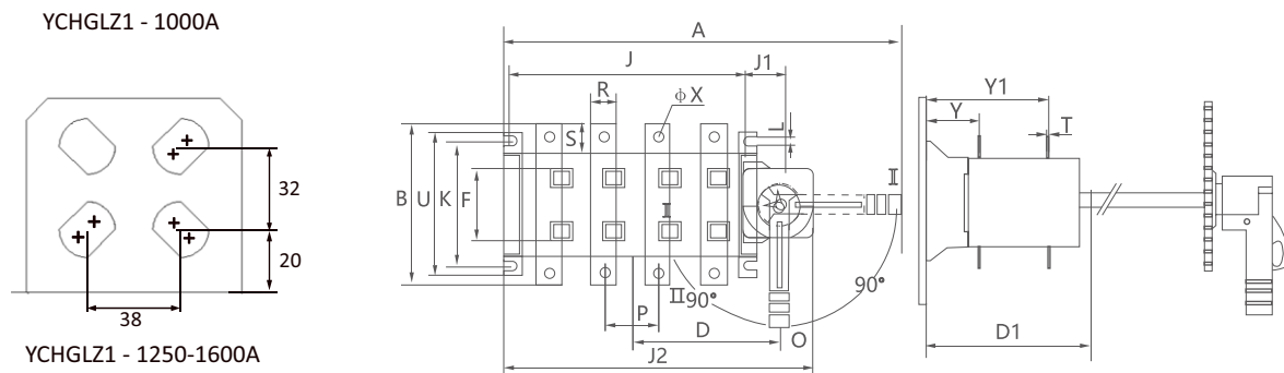
YCHGLZ1 160-1600A управление с дверцы шкафа
