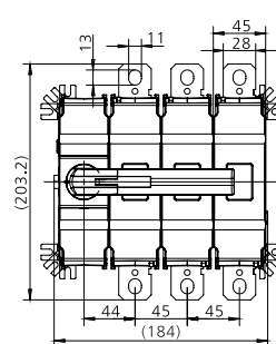
YCOT EHA B 630/630A 22
