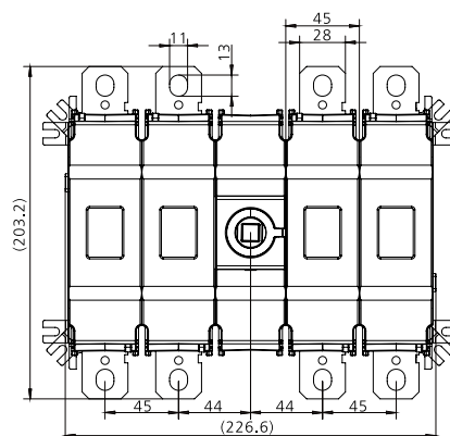
YCOT EHA C 630/800A 22
